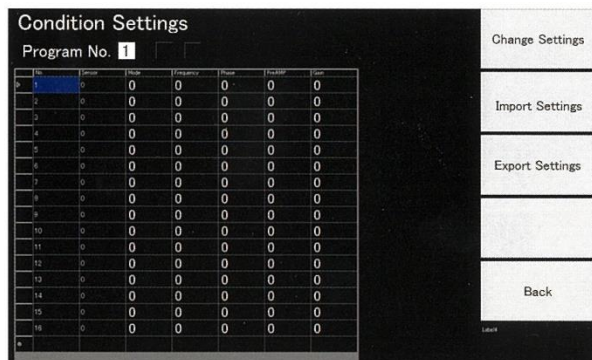
MSK-200の設定画面 一度の測定で16パターンの測定条件で測定できます。
